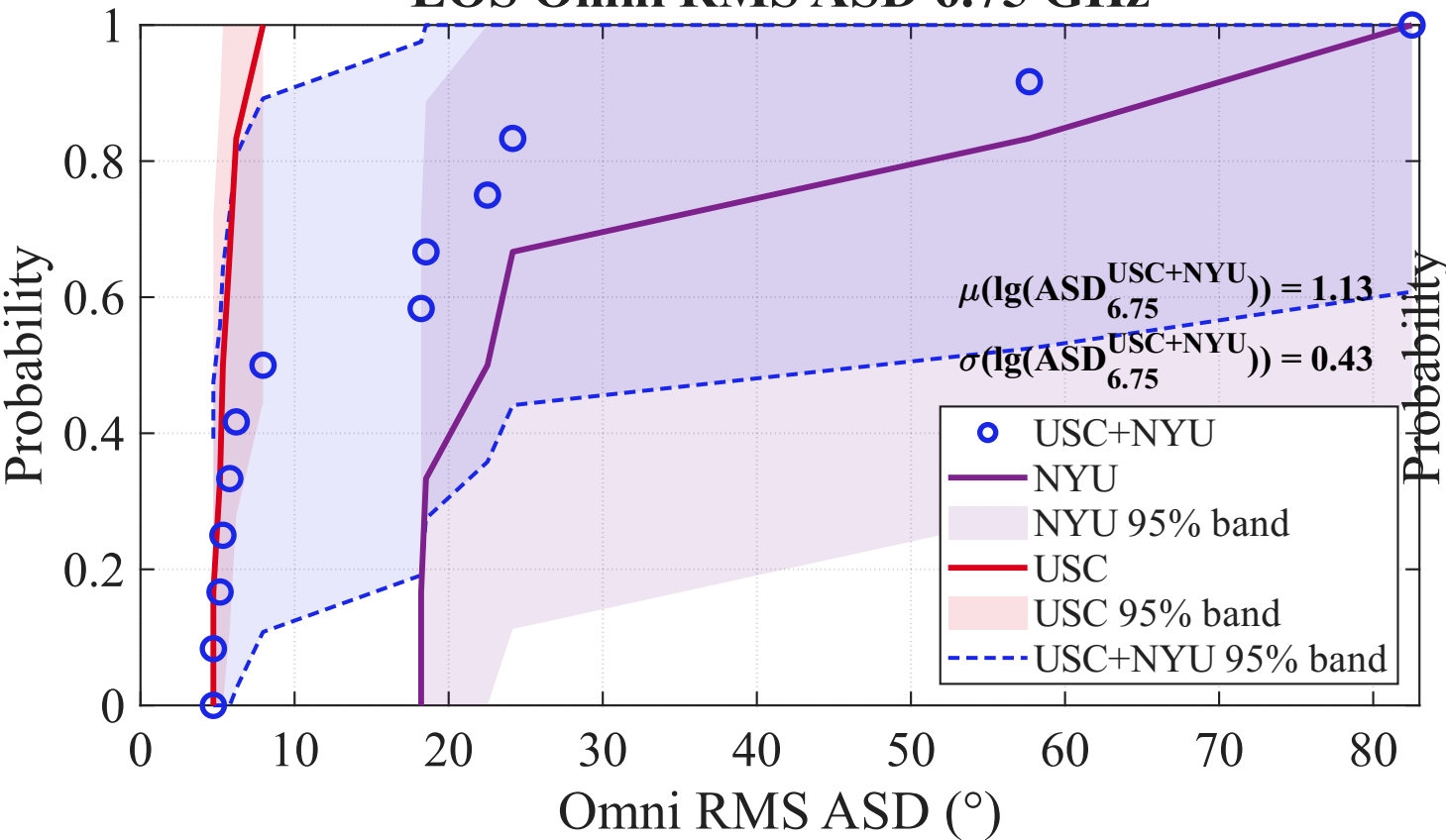
LOS Omni RMS ASD 6.75 GHz
