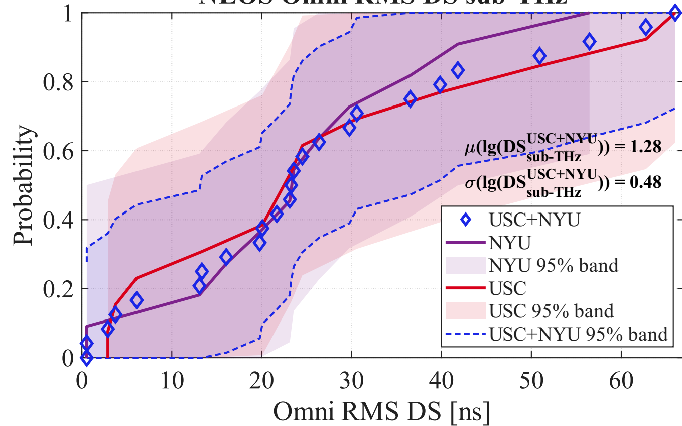
NLOS Omni RMS DS sub-THz
