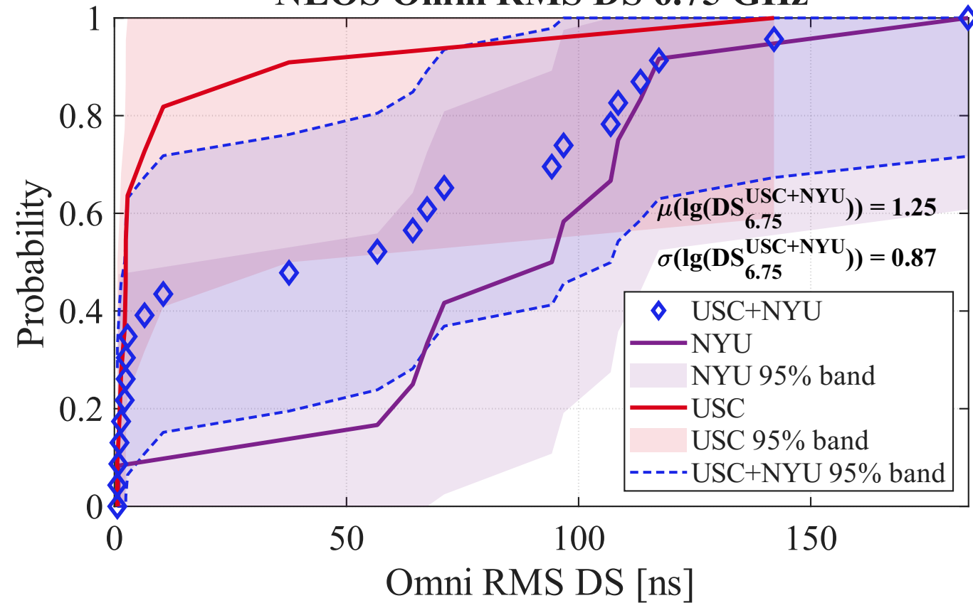
NLOS Omni RMS DS 6.75 GHz
