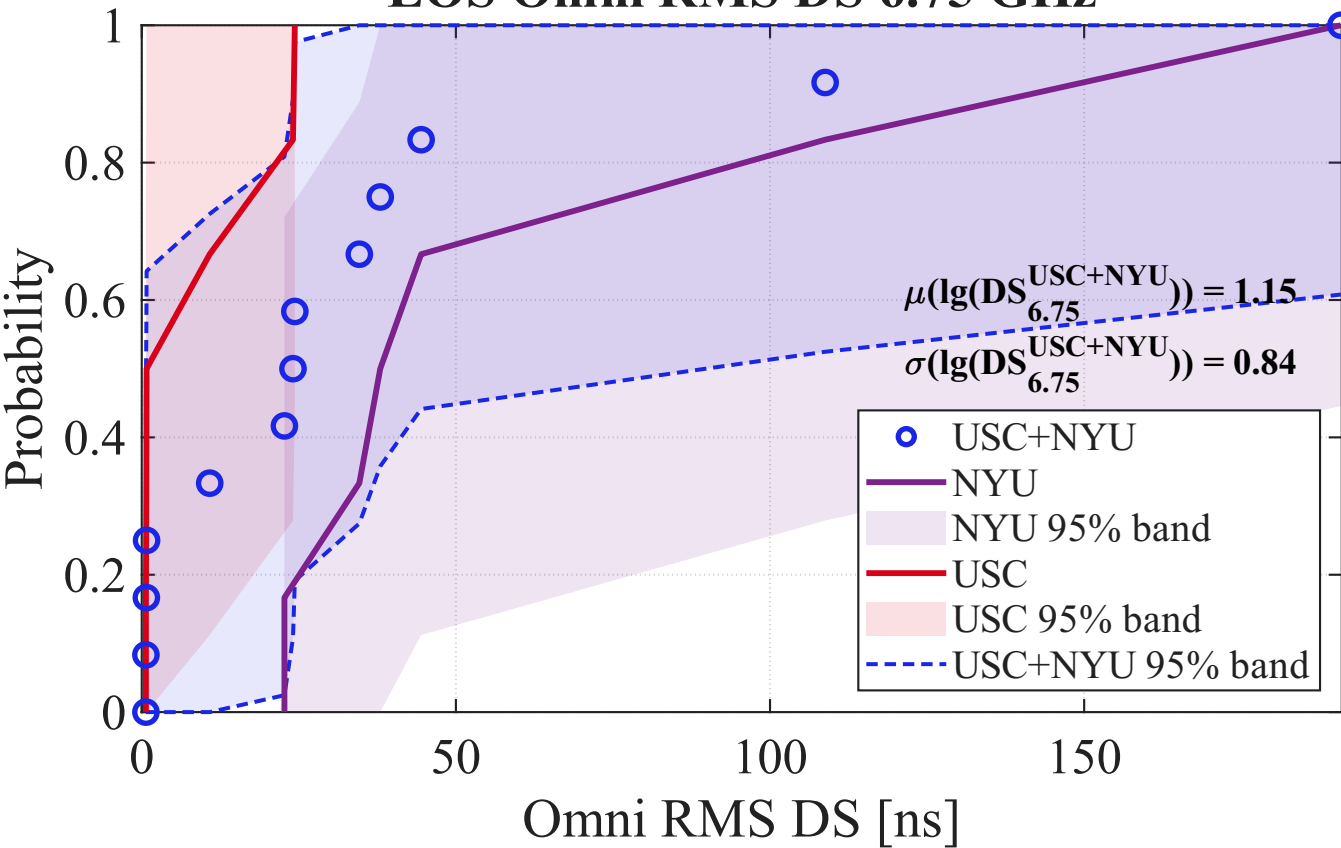
LOS Omni RMS DS 6.75 GHz
