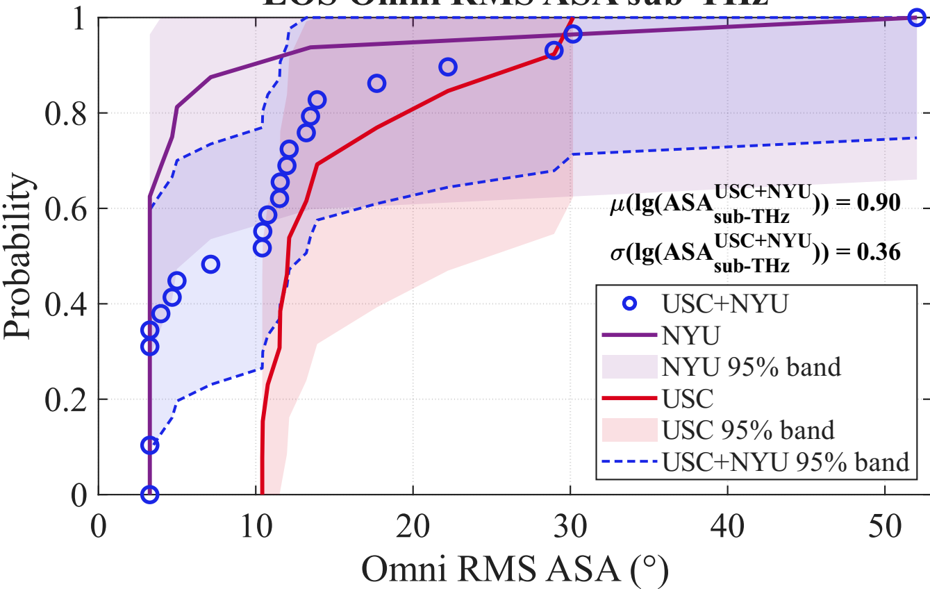
LOS Omni RMS ASA sub-THz
