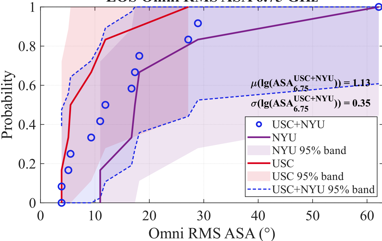
LOS Omni RMS ASA 6.75 GHz
