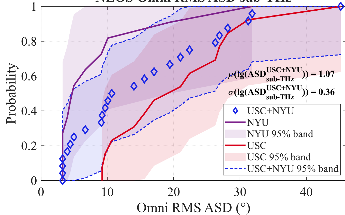
NLOS Omni RMS ASD sub-THz
