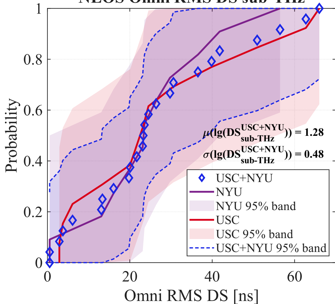
NLOS Omni RMS DS sub-THz
