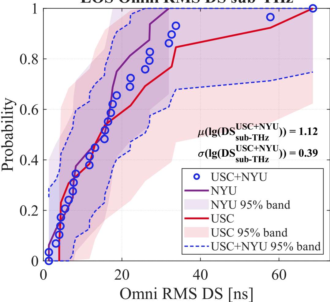
LOS Omni RMS DS sub-THz
