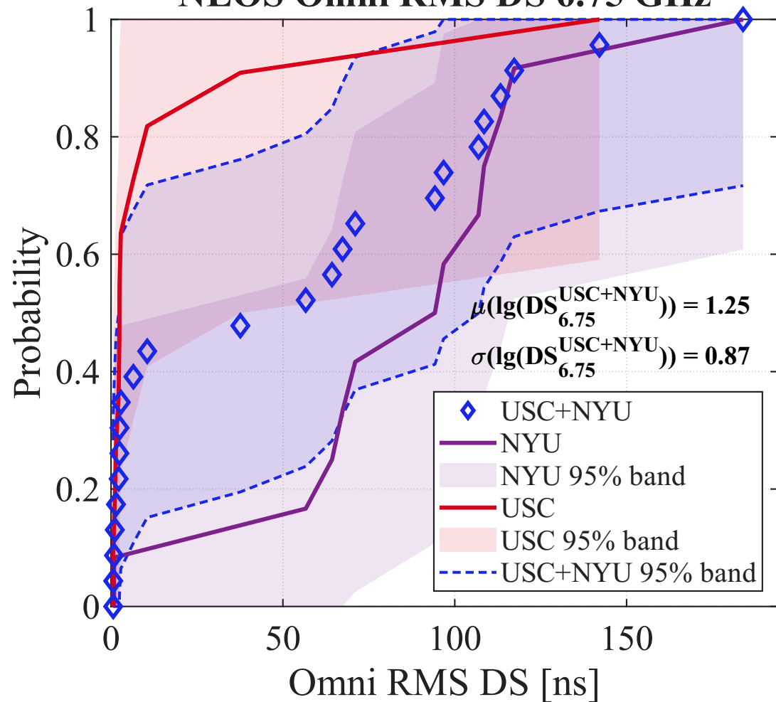
NLOS Omni RMS DS 6.75 GHz
