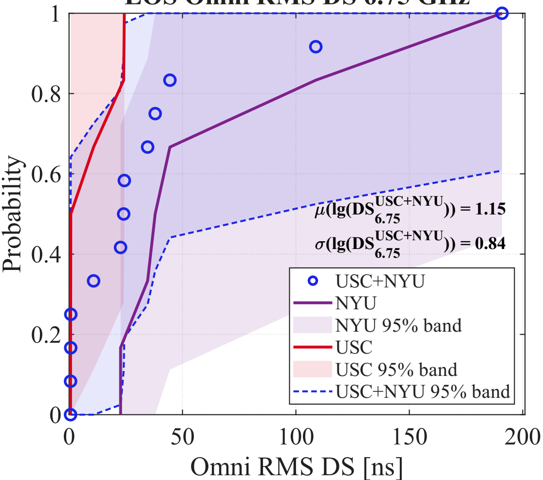
LOS Omni RMS DS 6.75 GHz
