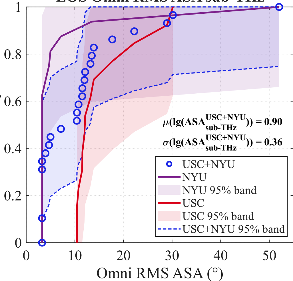
LOS Omni RMS ASA sub-THz
