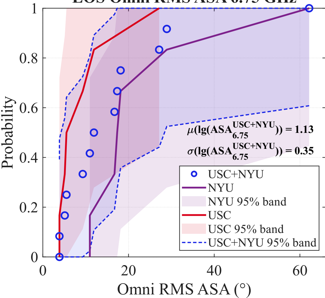
LOS Omni RMS ASA 6.75 GHz
