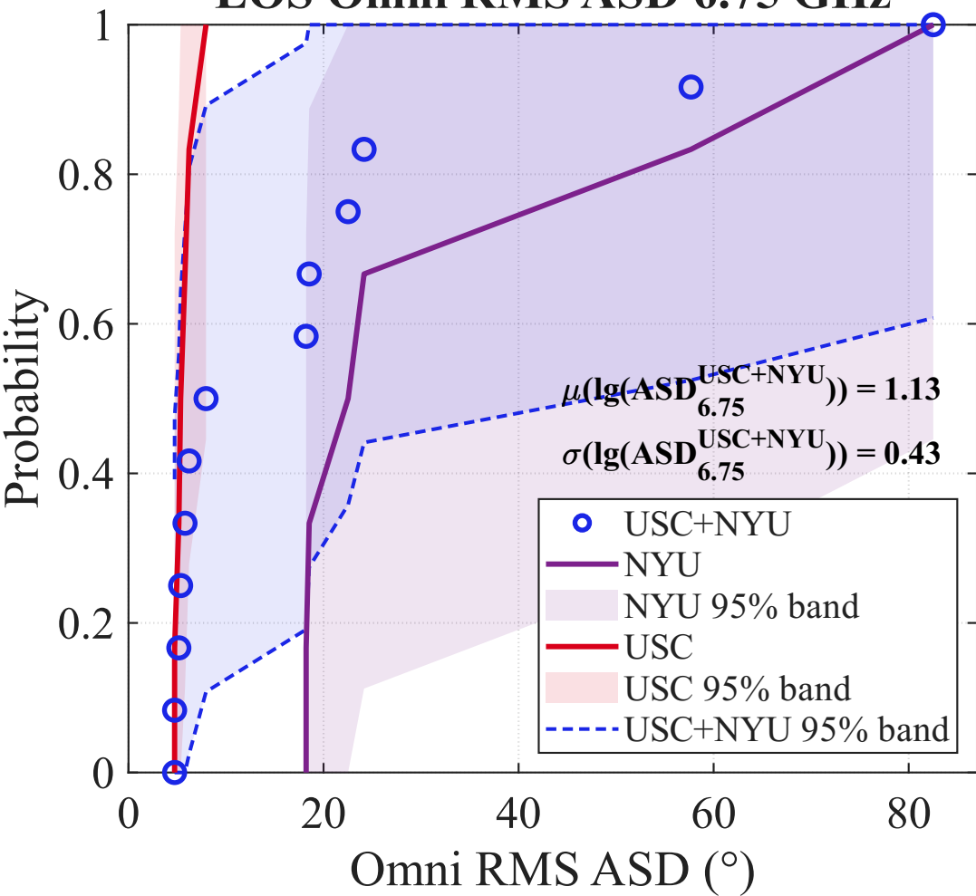
LOS Omni RMS ASD 6.75 GHz
