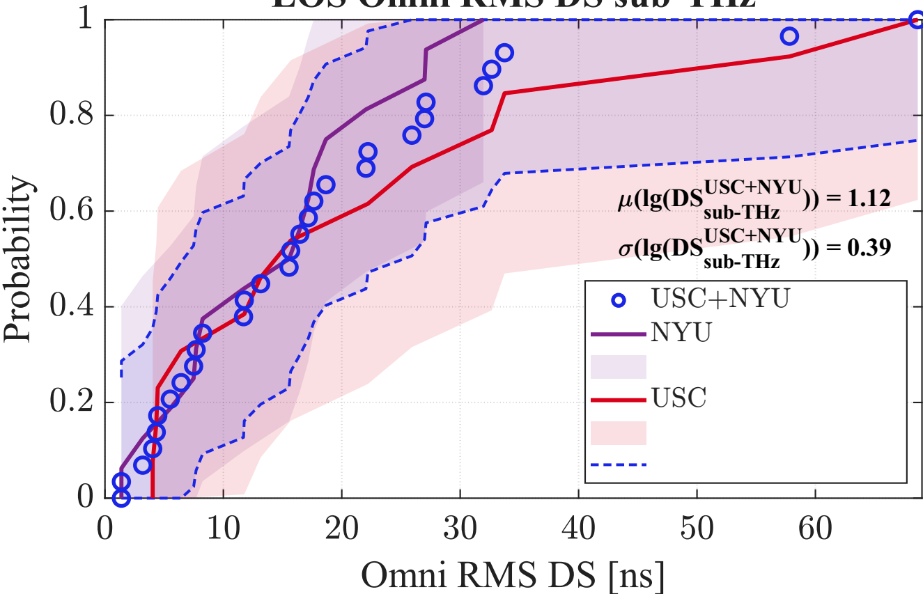
LOS Omni RMS DS sub-THz
