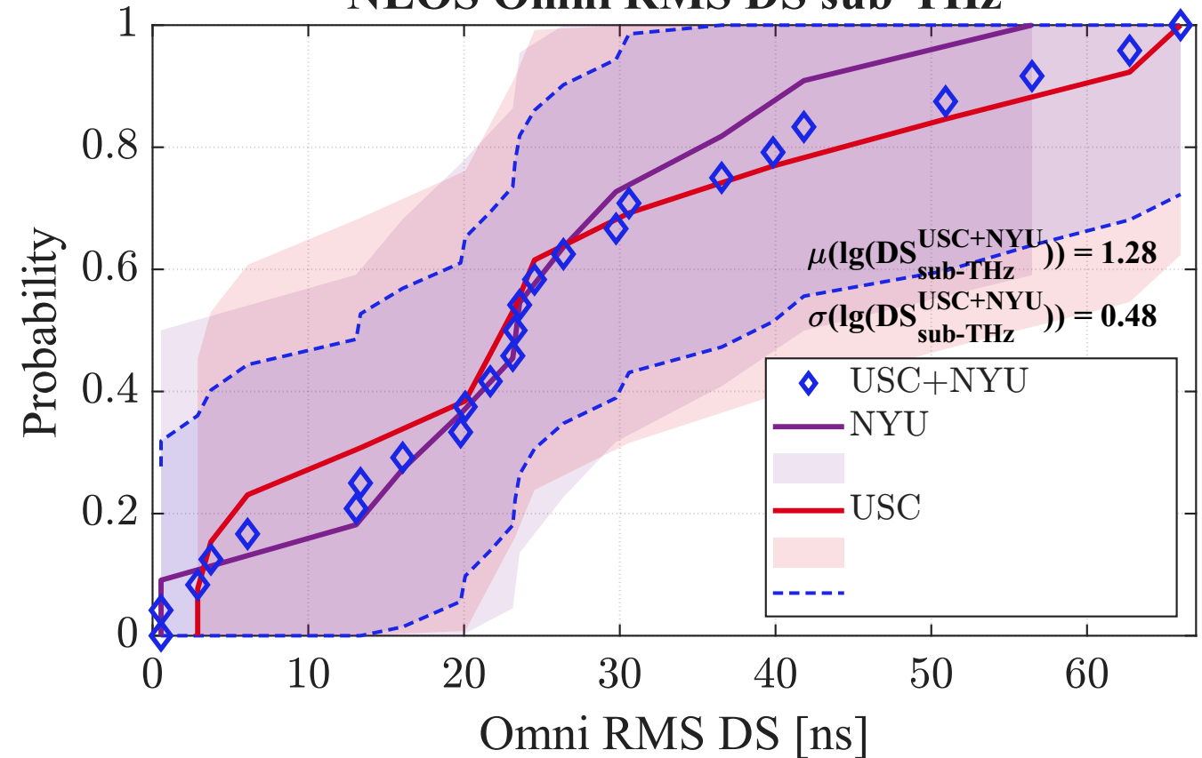
NLOS Omni RMS DS sub-THz
