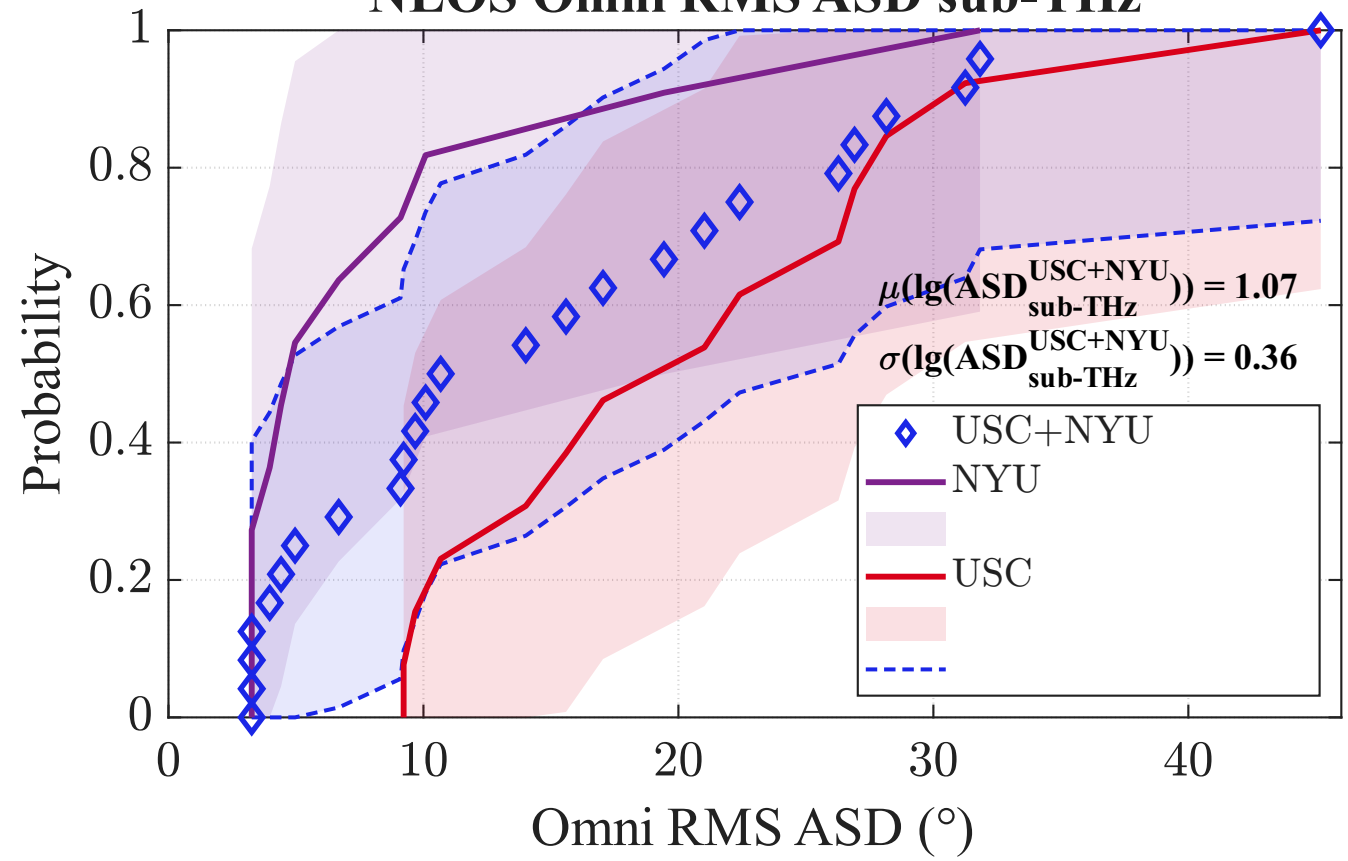
NLOS Omni RMS ASD sub-THz
