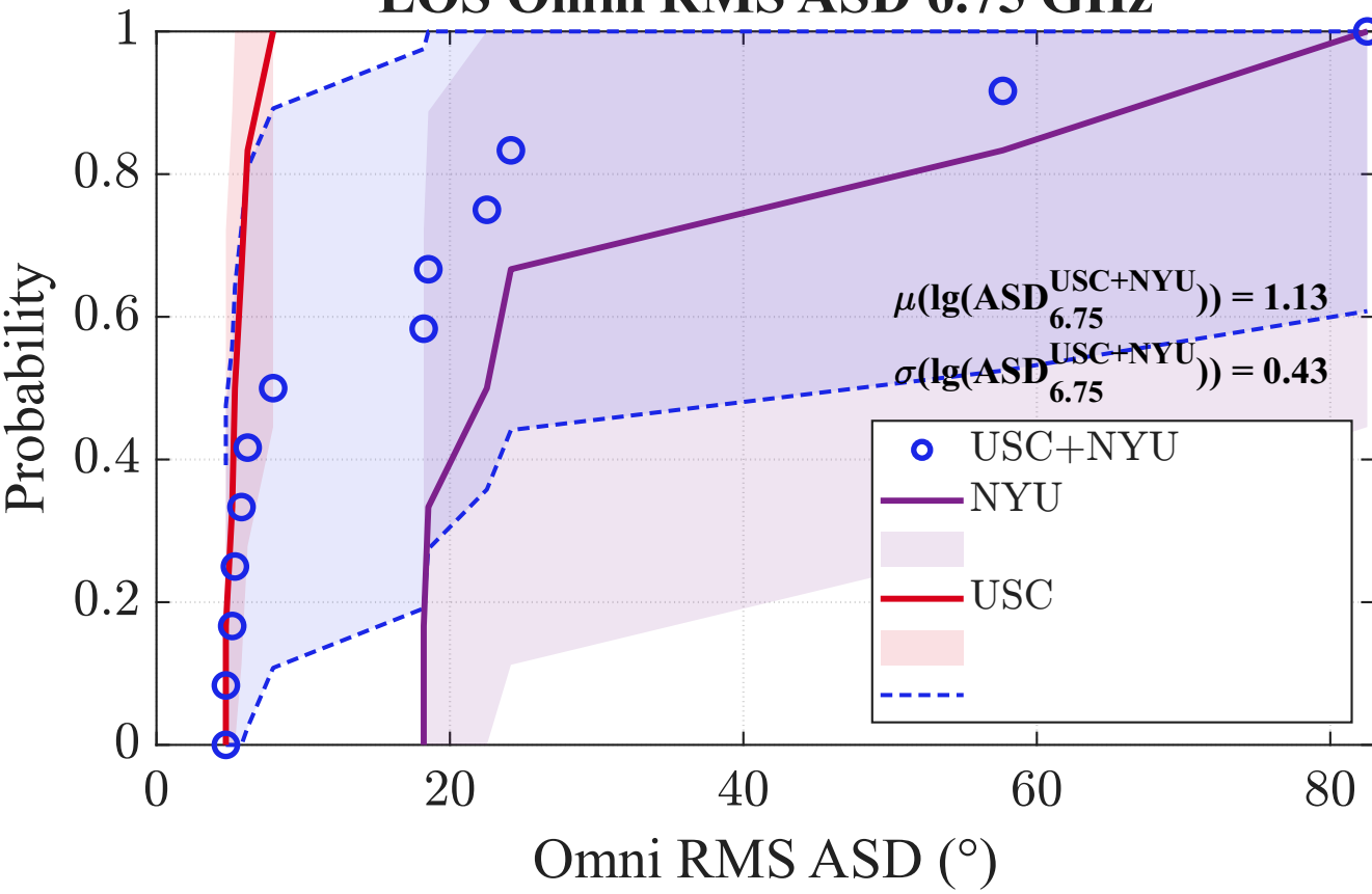
LOS Omni RMS ASD 6.75 GHz
