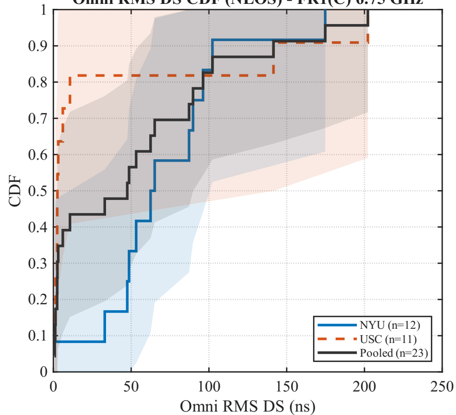
Omni RMS DS CDF (NLOS) - FR1(C) 6.75 GHz
