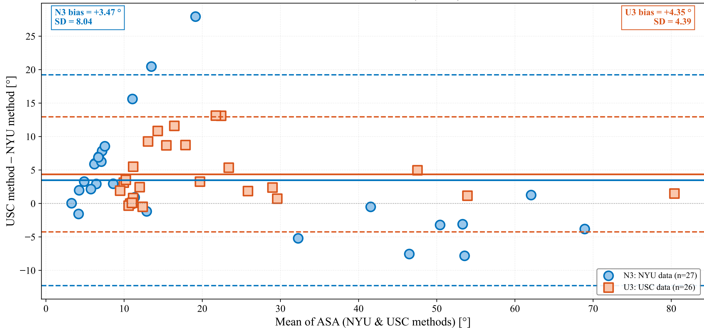
Bland-Altman: Omni ASA (sub-THz)
