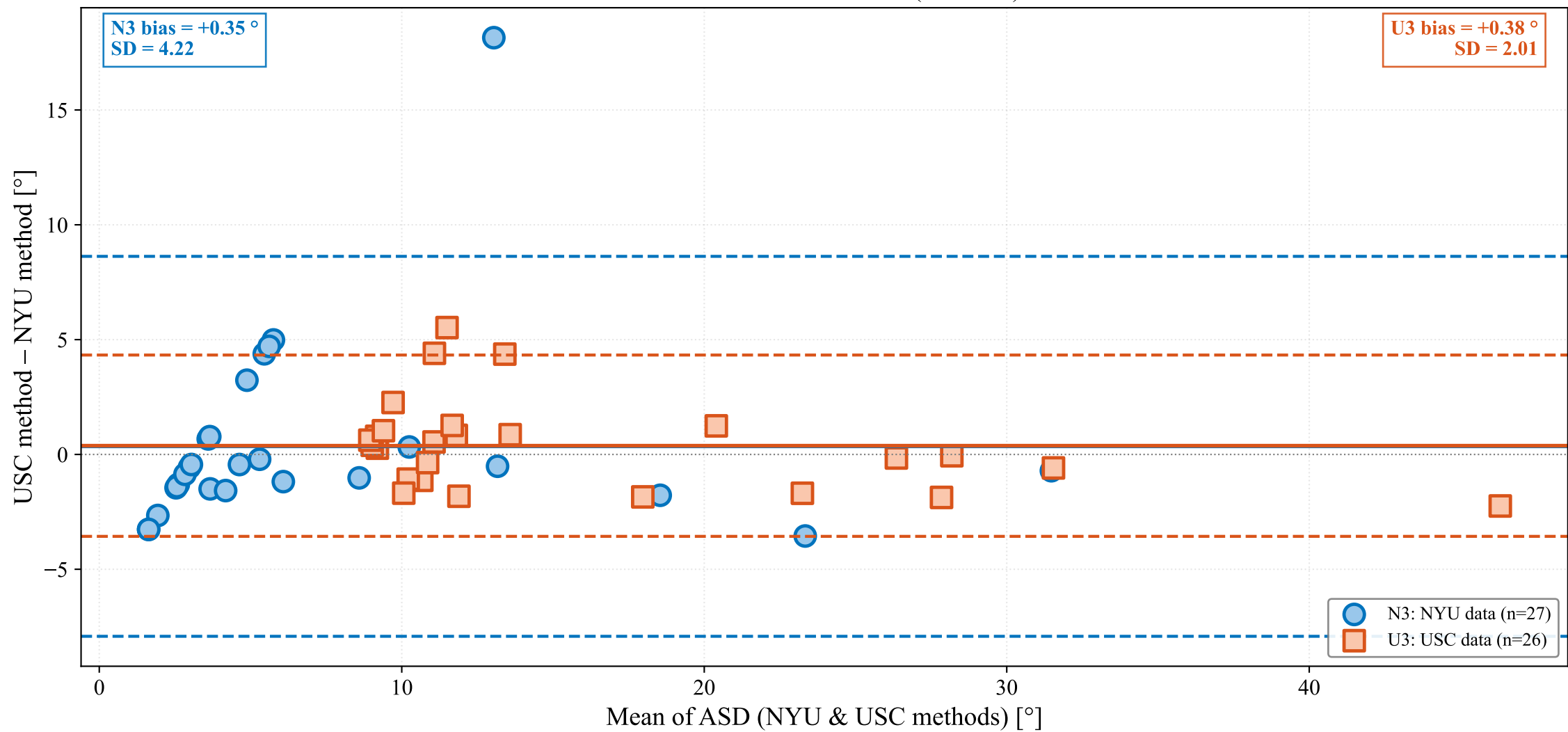
Bland-Altman: Omni ASD (sub-THz)
