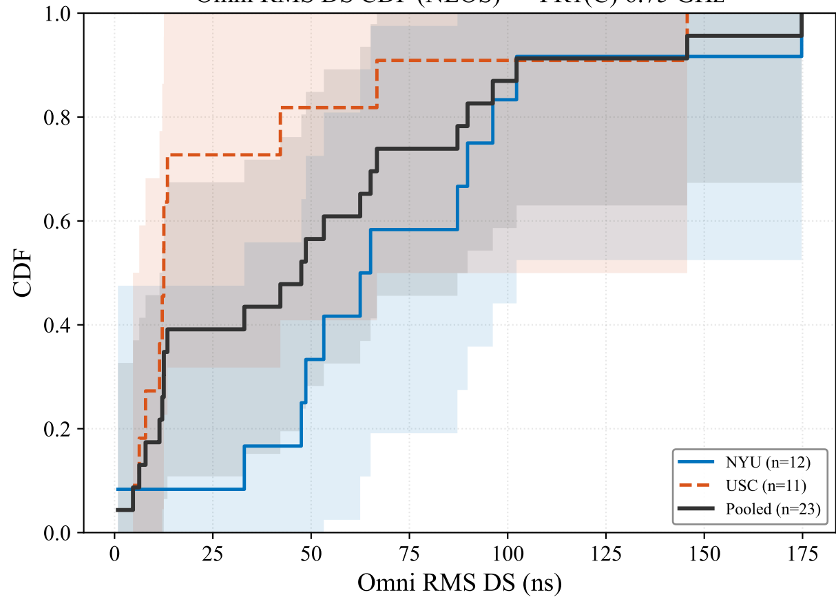
Omni RMS DS CDF (NLOS) — FR1(C) 6.75 GHz
