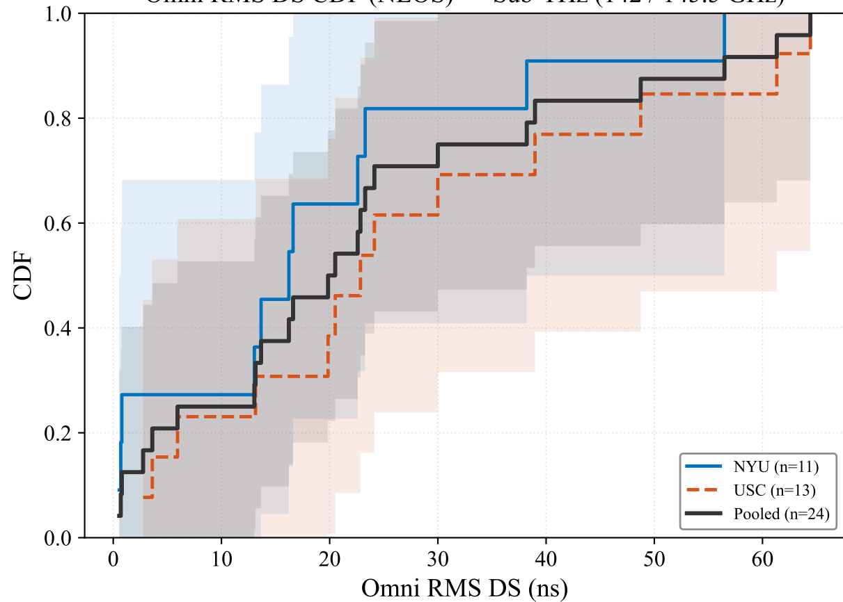
Omni RMS DS CDF (NLOS) — Sub-THz (142 / 145.5 GHz)
