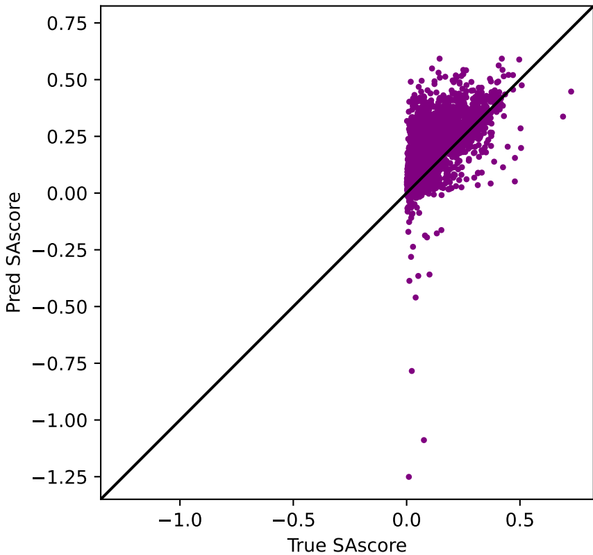
SA score (Pearson r = 0.591 )
