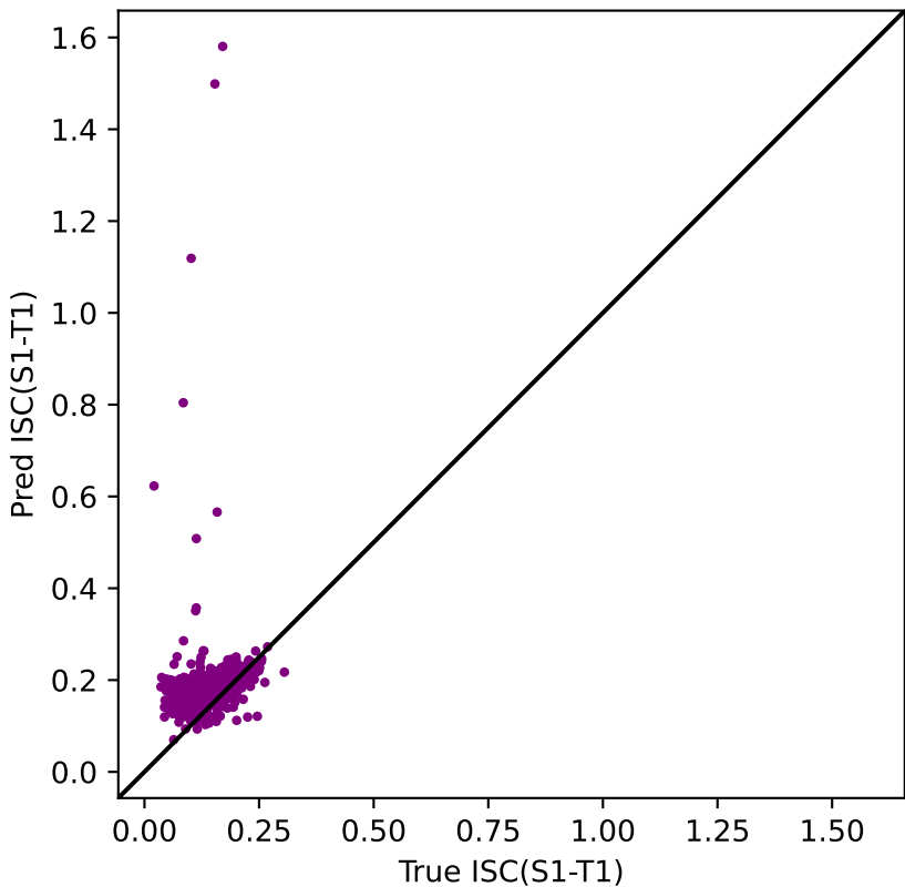
ISC(S1-T1) (Pearson r = 0.119 )
