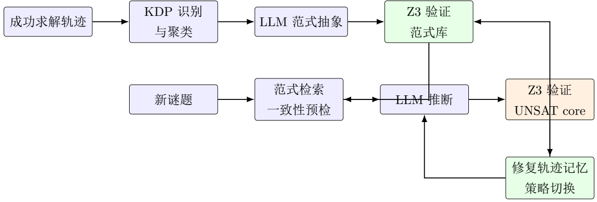
图 1: PRISM 的离线范式提炼与在线修复记忆框架。 离线 （上行）：成功求解轨迹经 KDP 识别、跨轨迹聚类、LLM 抽象和 Z3 三重验证，提炼为可复用范式库（约 40:1 压缩比）。 在线 （下行）：新谜题的推断步骤由范式引导并经 Z3 验证；若返回 UNSAT，系统提取 UNSAT core 进行归因，记录至类型化修复记忆，并在检测到停滞或循环时触发 L1-L4 策略切换。
