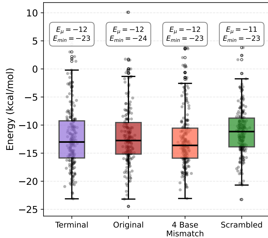
Van der Waals Energy
