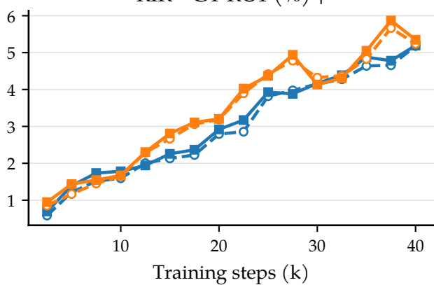
RIR→GT R@1 (%) ↑
