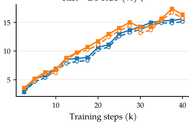
RIR→GT R@5 (%) ↑
