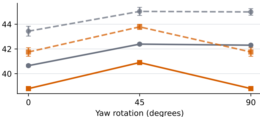
EDT error (ms) \downarrow
