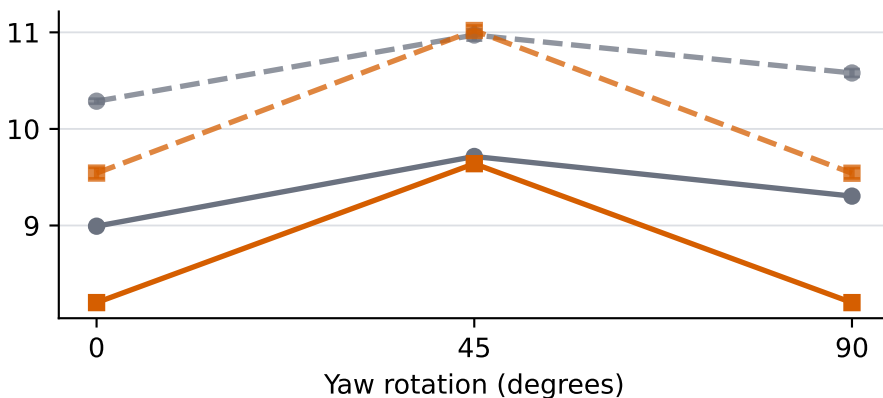
T60 error (%) \downarrow
