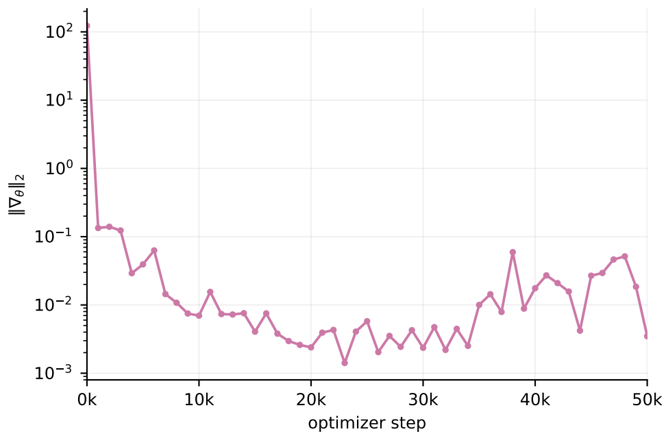
Gradient norm
