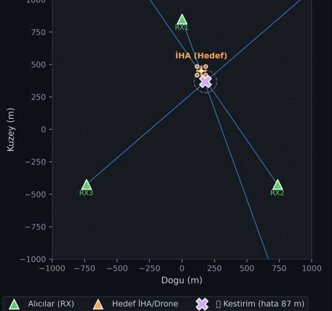
4.5 Konum Belirleme — LOB Kesişimi (Triangulation)
