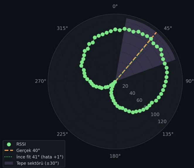
4.4 Yön Bulma (DF) — Dönen Yönlü Anten, 360° Geniş Tarama Tepe: 40° (hata +0°) | İnce: 41° (hata +1°)
