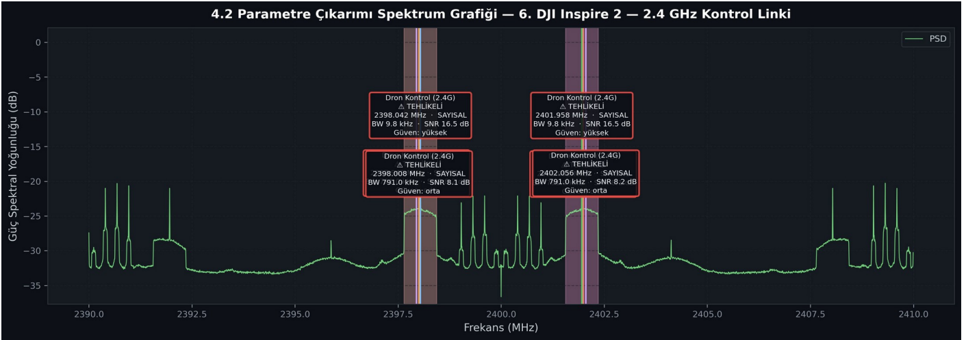
Parametre çıkarımı — CF / BW / SNR ve cihaz sınıflandırması etiketli spektrum
