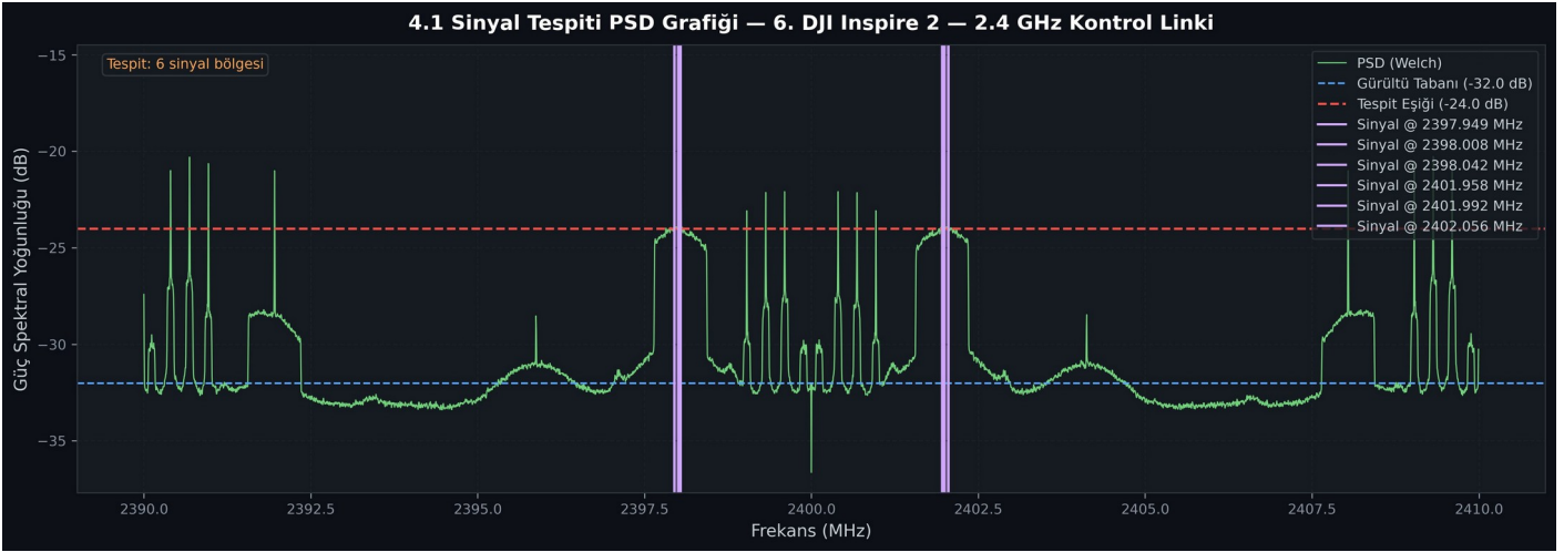
Sinyal tespiti — Welch PSD, gürültü tabanı, adaptif eşik, tespit bölgeleri
