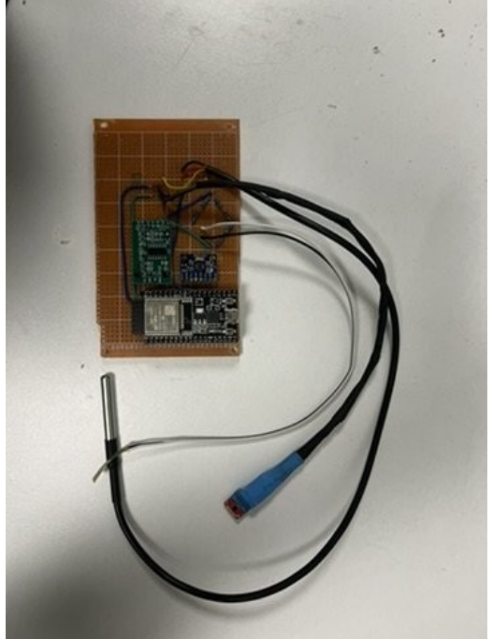
Elle lehimlenen ESP32 sensör devresi – arka (bağlantı hatları) ve ön (sıcaklık sensörü, konektör) görünüm
