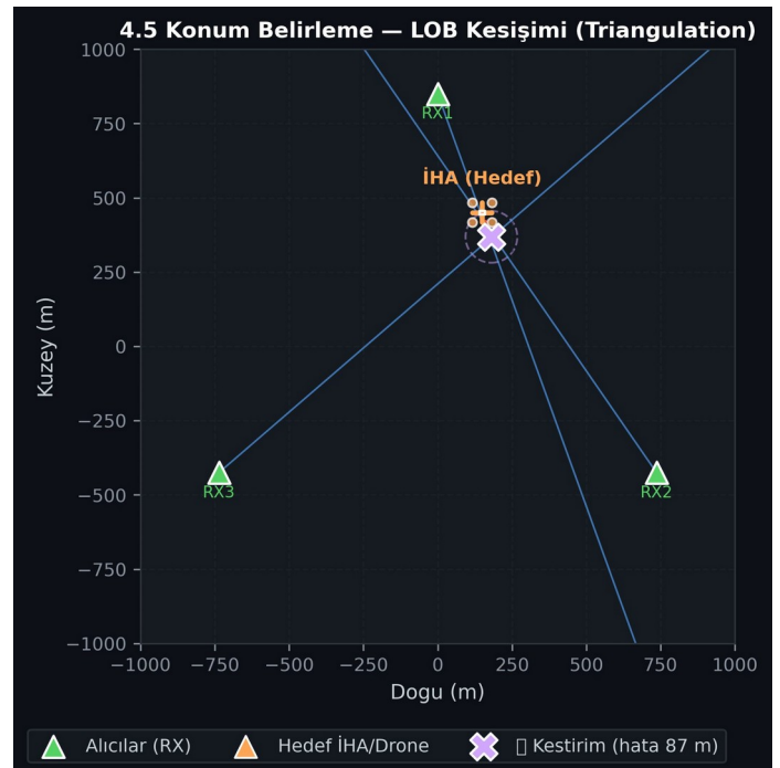
Sağ: LOB kesişimiyle konum belirleme
