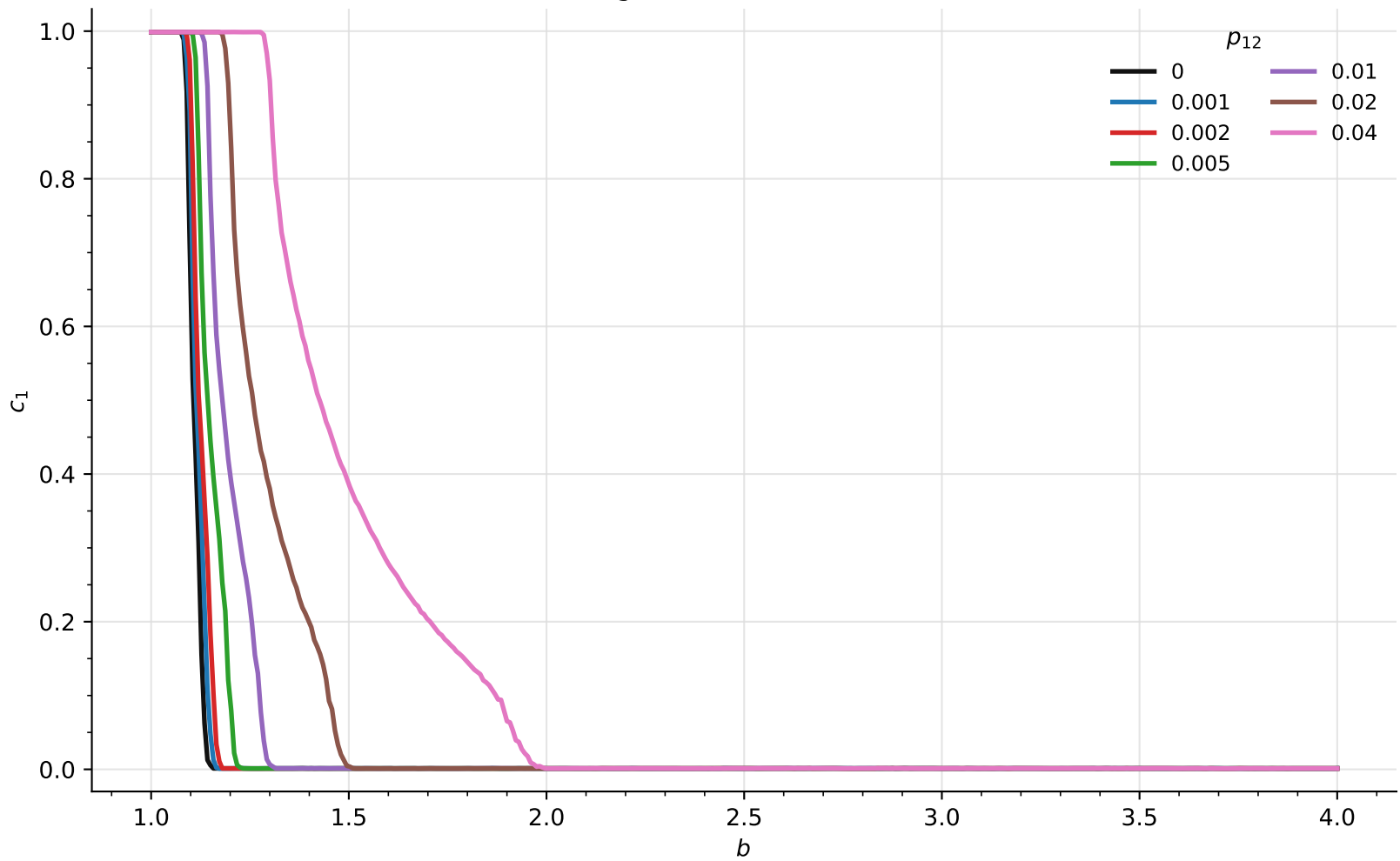
Fig. 4 Fermi, beta=10
