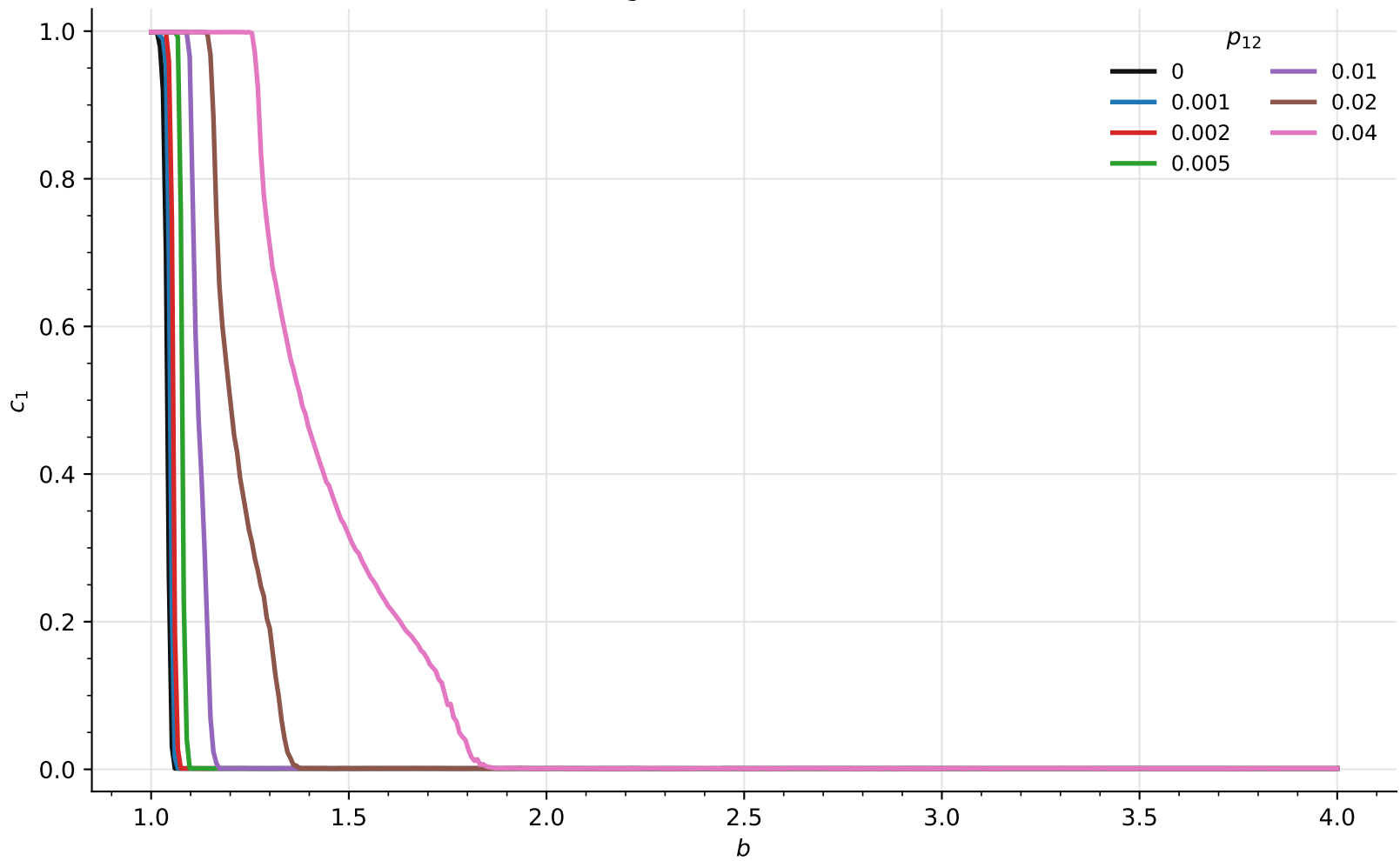
Fig. 4 Fermi, beta=5
