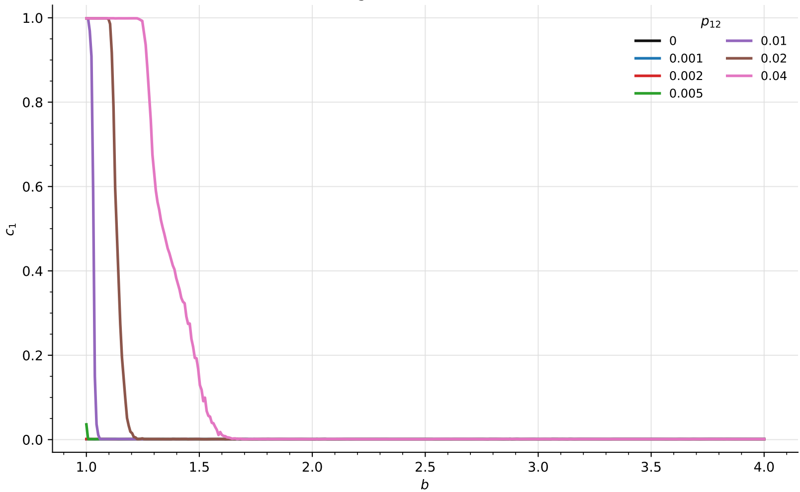
Fig. 4 Fermi, beta=1
