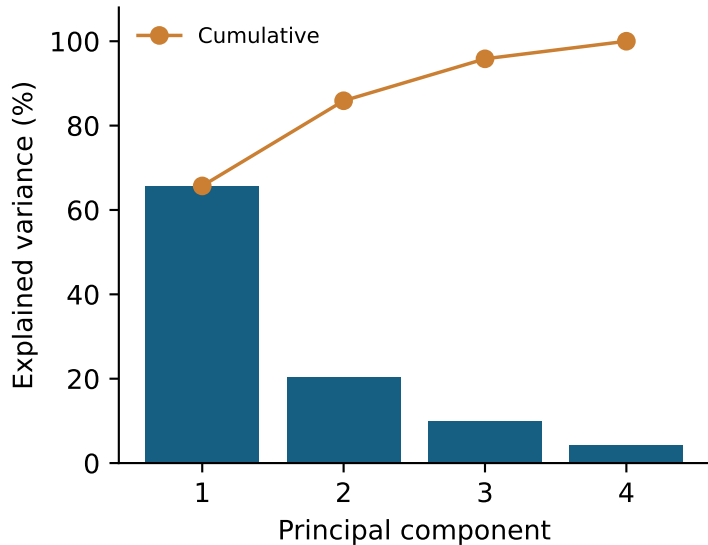
(b) Covariance eigenvalues
