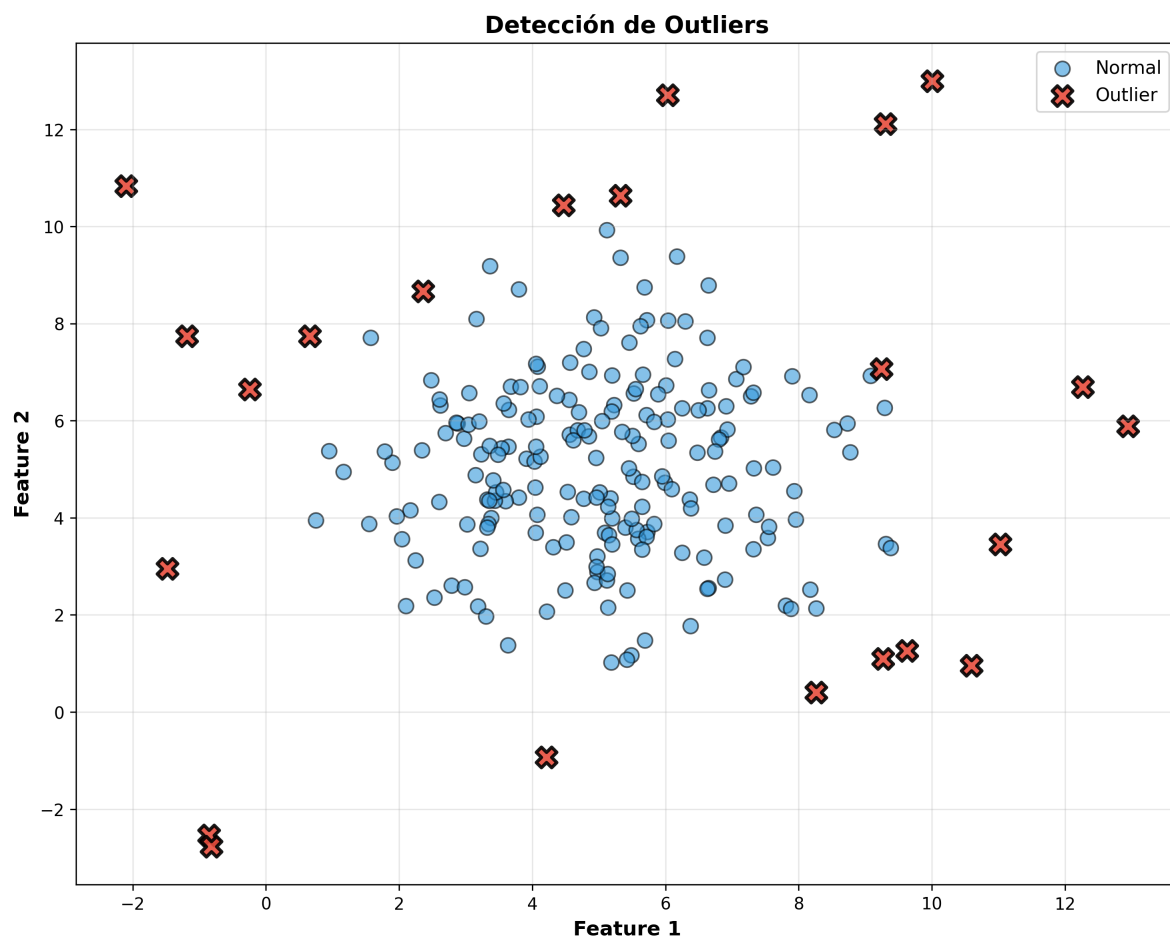
Figura 1: Visualización de outliers
