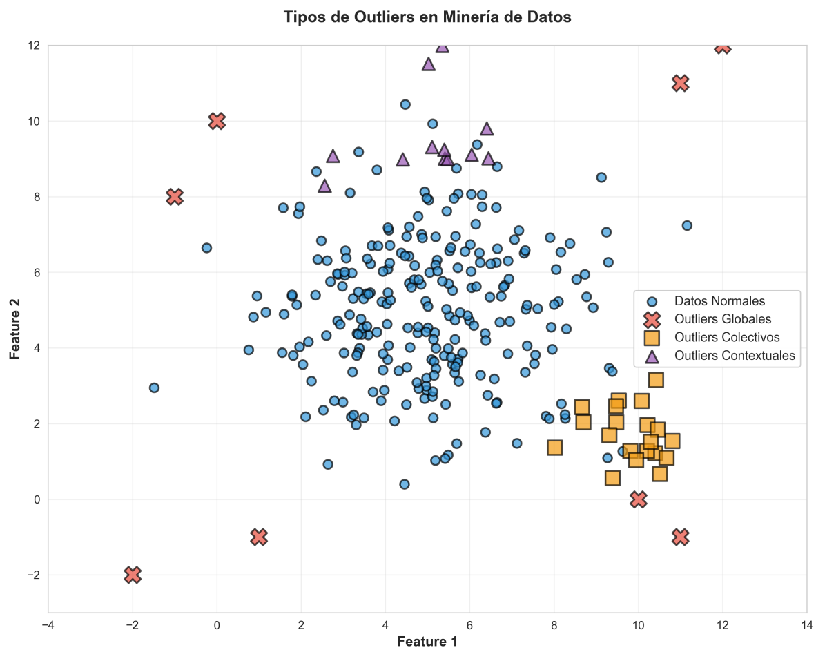
Figura 1: Visualización de tipos de Outliers
