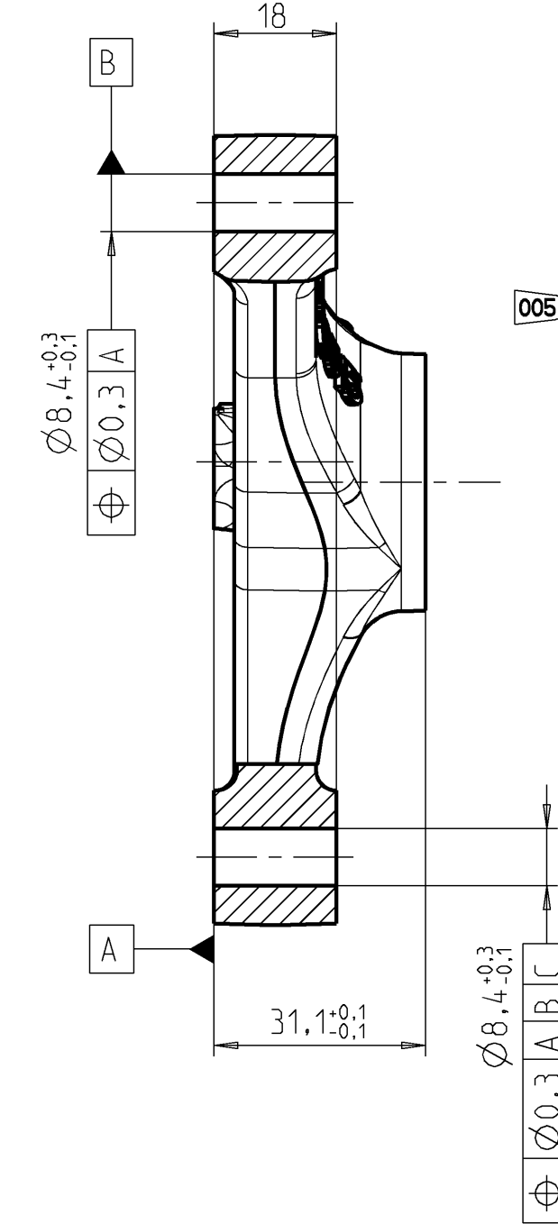
SCHNITT SECTION COUPE
