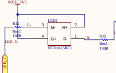
LED指示灯
