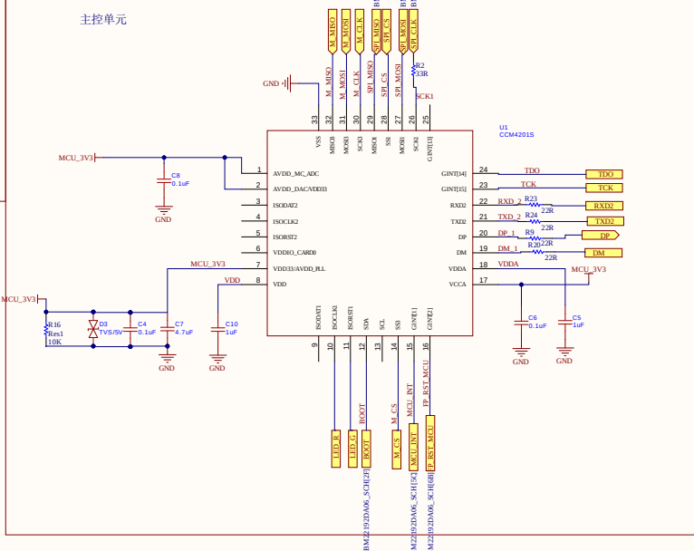
主控单元
