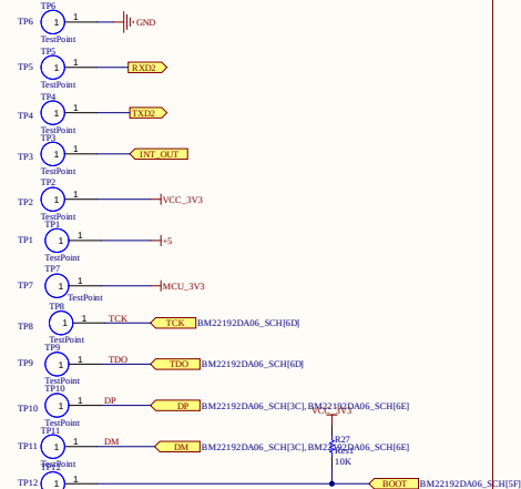
测试及烧录点
