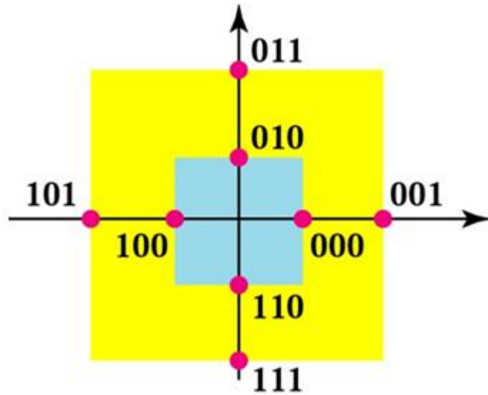
8QAM
