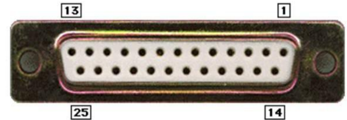
DB-25 Female (DTE side)
