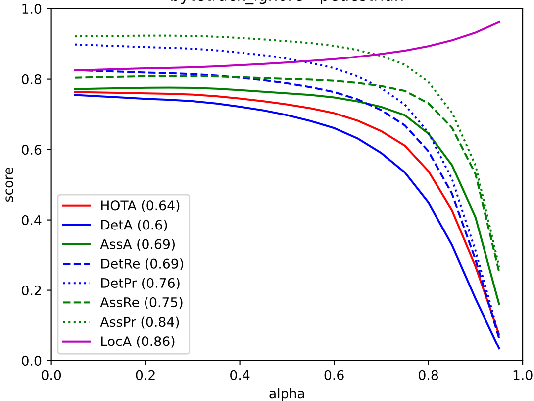
bytetrack_ignore - pedestrian
