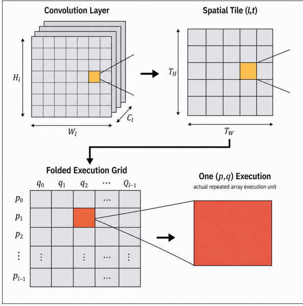
图 2 固定规模阵列上的折叠映射。从卷积层选取空间分块后，阵列沿规约轮次 p 和输出通道块 q 形成执行网格；其中一个 (p, q) 单元对应一次实际阵列执行。
