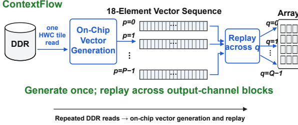
图 1 ContextFlow 的两项问题动机。片上向量生成与重放减少跨输出通道块的重复输入，上下文流水通过预取、部分和反馈与直接切换缩短相邻执行边界。
