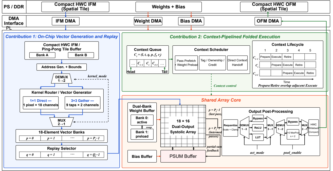
图 3 ContextFlow 总体架构与执行模型。外部保持紧凑 HWC 张量，两项核心机制在固定阵列前后组织片上复用和跨轮次重叠。
