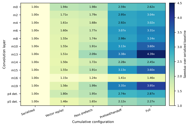
图9 五级配置相对串行基线的逐层累计加速。每个单元格为 T_{\text{serialized}}/T_{\text{configuration}} ，数值越大表示累计收益越高。
