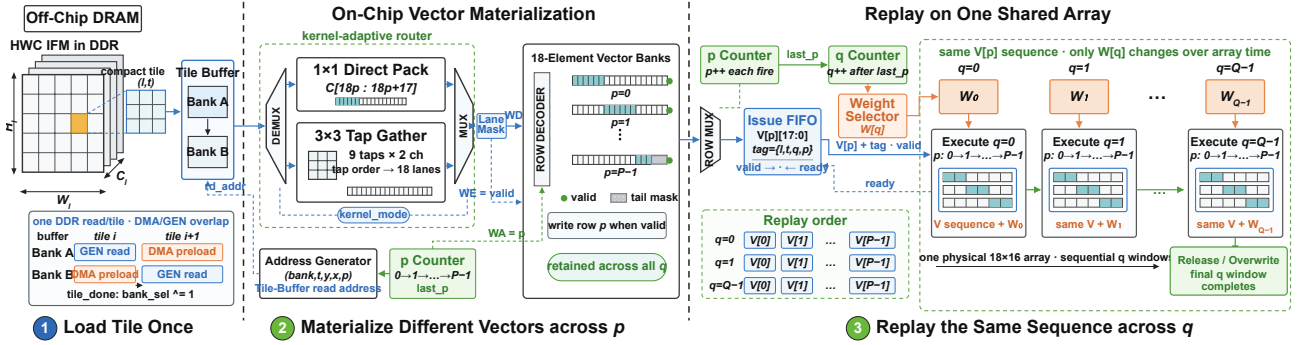
图 4 HWC 分块的片上向量生成与跨输出通道块重放机制。紧凑输入分块只读取一次；片上路由器按规约轮次 p 生成并缓存 18 元素向量，不同输出块 q 在同一物理阵列上重放整套向量序列，并在最后一个读取者完成后释放缓存。
