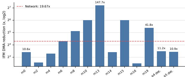
图 7 片上向量生成与重放相对串行输入方式的逐层 IFM DMA 降低倍数。纵轴采用以 2 为底的对数刻度，虚线表示完整网络的 19.67 倍降低。
