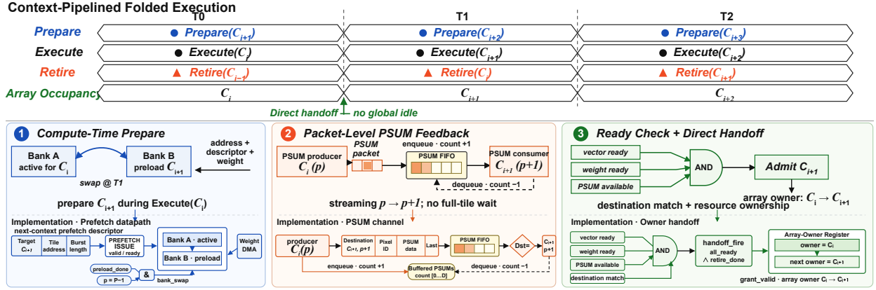
图5 面向折叠执行的上下文流水时序与三项实现机制。相邻上下文的准备、计算和退休在阵列独占约束下重叠；计算期预取、数据包级部分和反馈及就绪检查支持直接切换。
