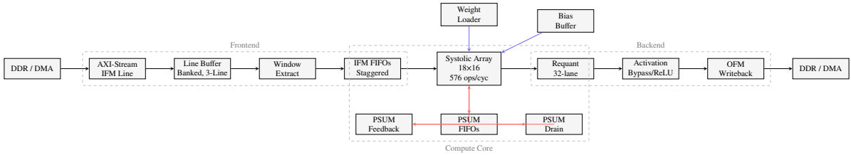
图 3.1 加速器整体架构框图
