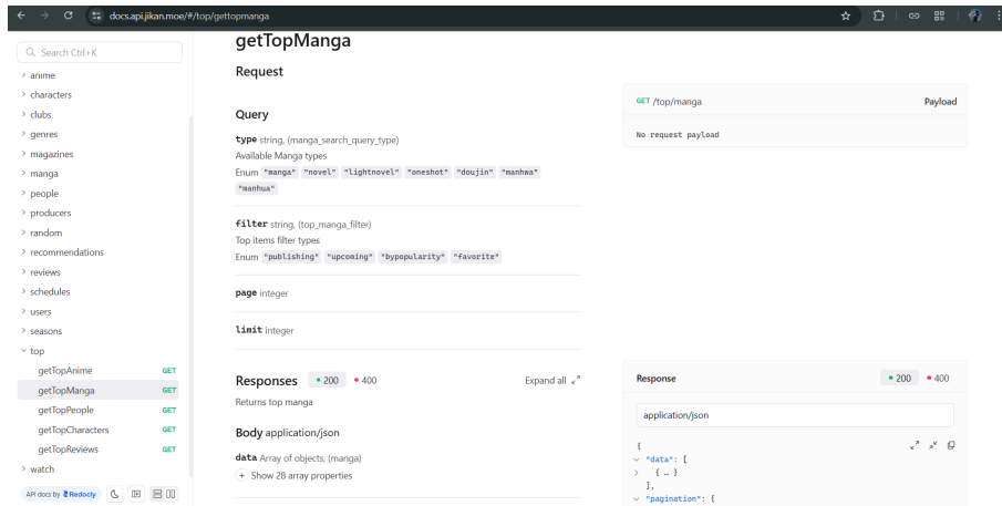
Gambar 2: Dokumentasi Jikan API
