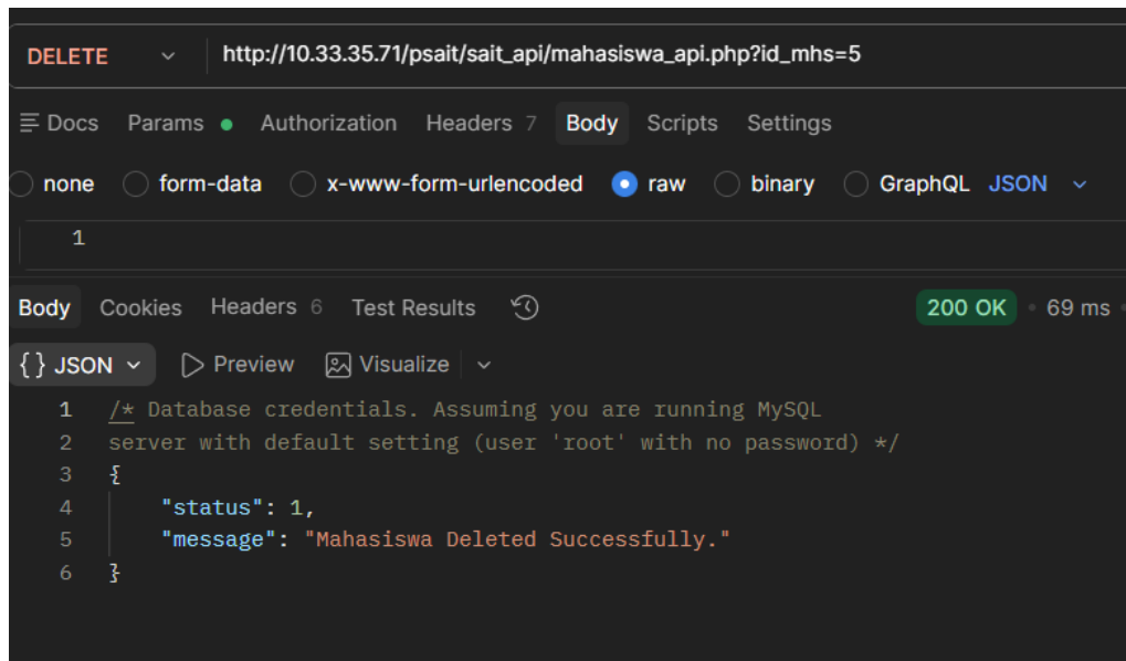
Gambar 5: Hasil pengujian REST API dengan Http Method DELETE
