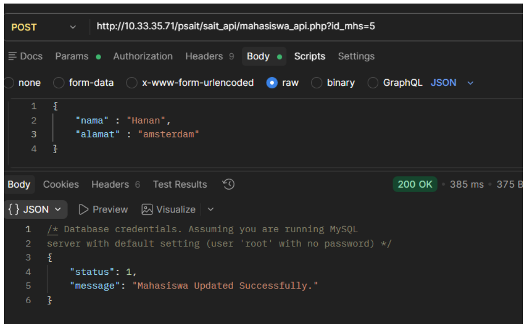
Gambar 4: Hasil pengujian REST API dengan Http Method POST untuk memperbarui data
