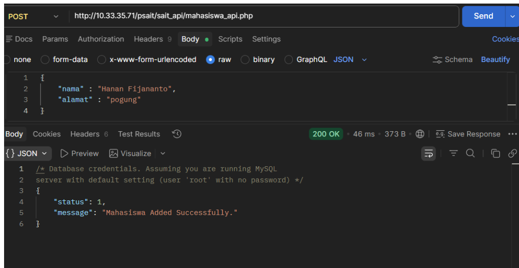
Gambar 3: Hasil pengujian REST API dengan Http Method POST
