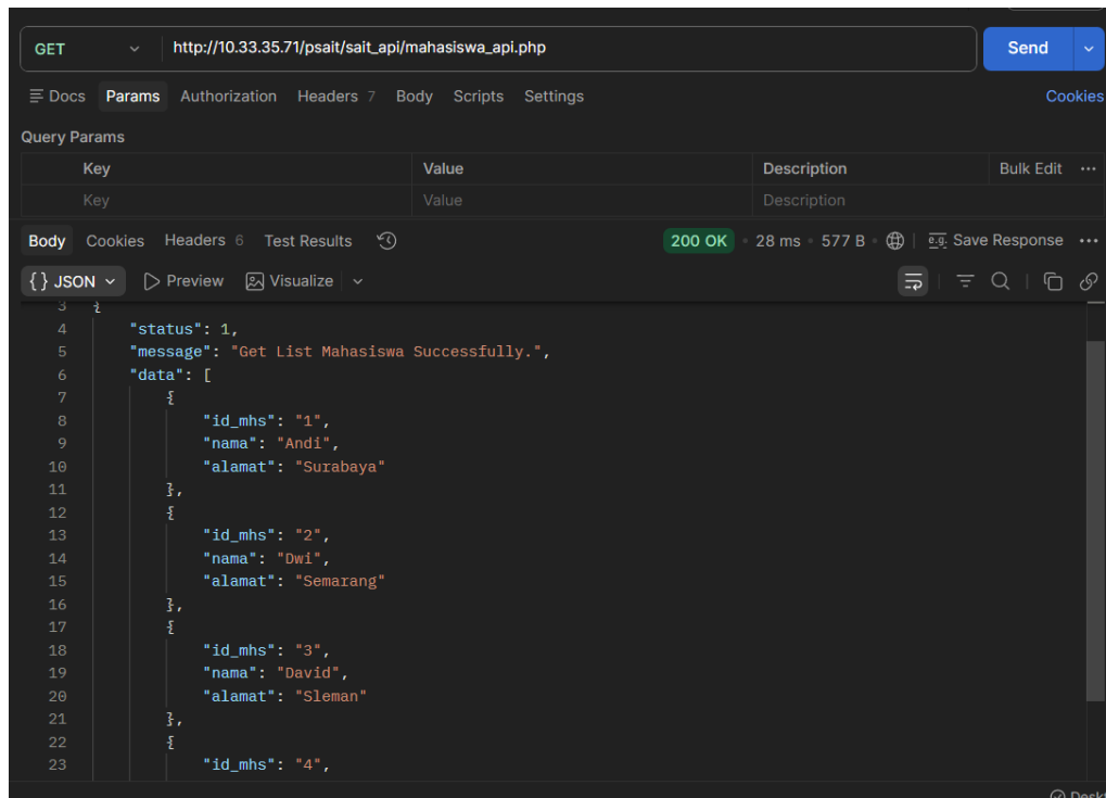
Gambar 2: Hasil pengujian REST API dengan Http Method GET
