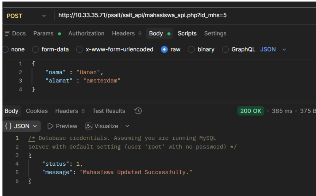
Figure 3: Hasil pengujian REST API dengan Http Method POST untuk memperbarui data
