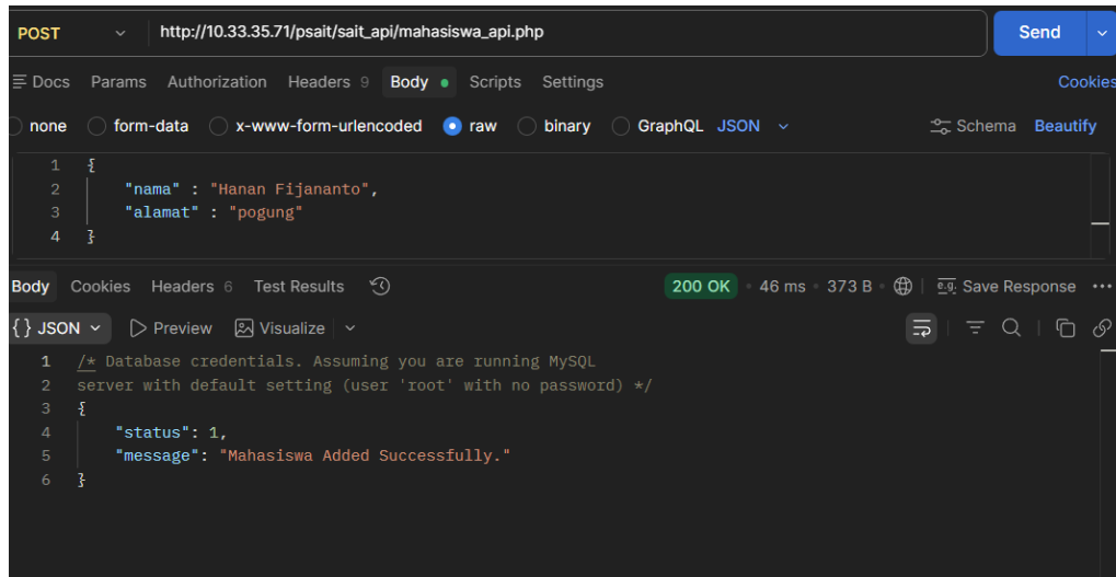
Figure 2: Hasil pengujian REST API dengan Http Method POST
