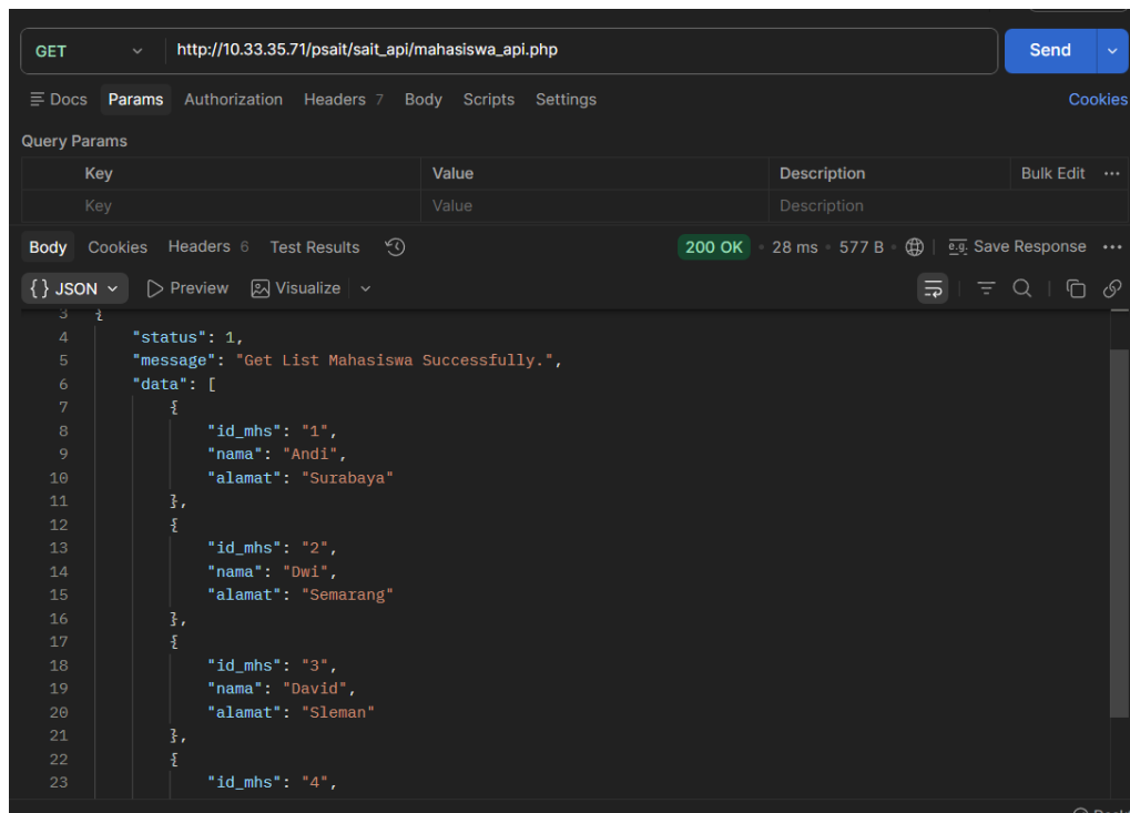
Figure 1: Hasil pengujian REST API dengan Http Method GET
