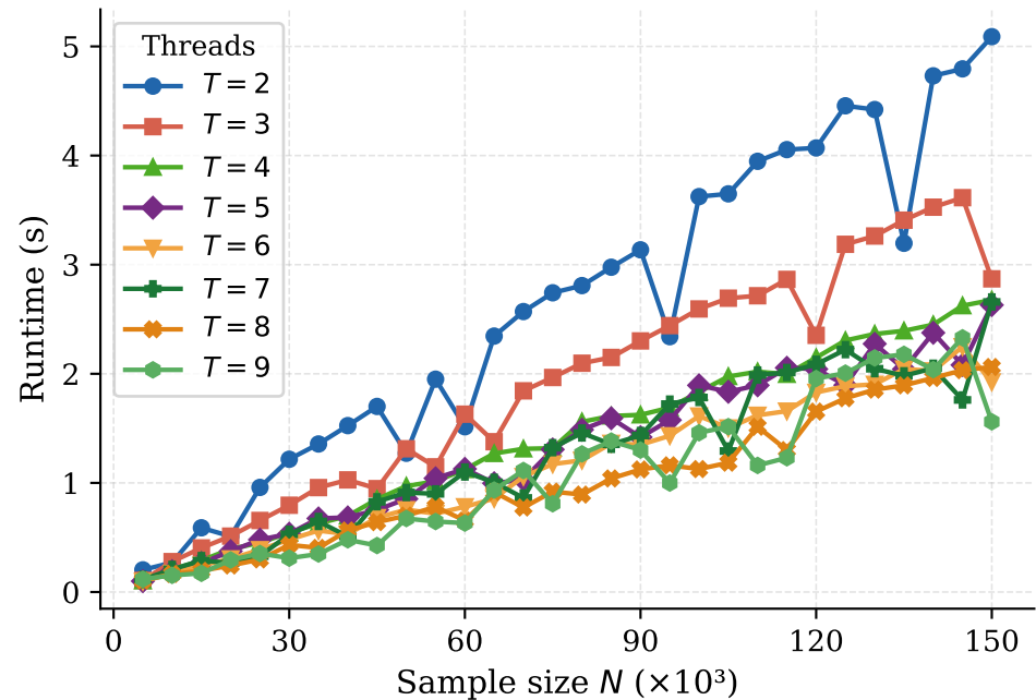
Gradient ascent
