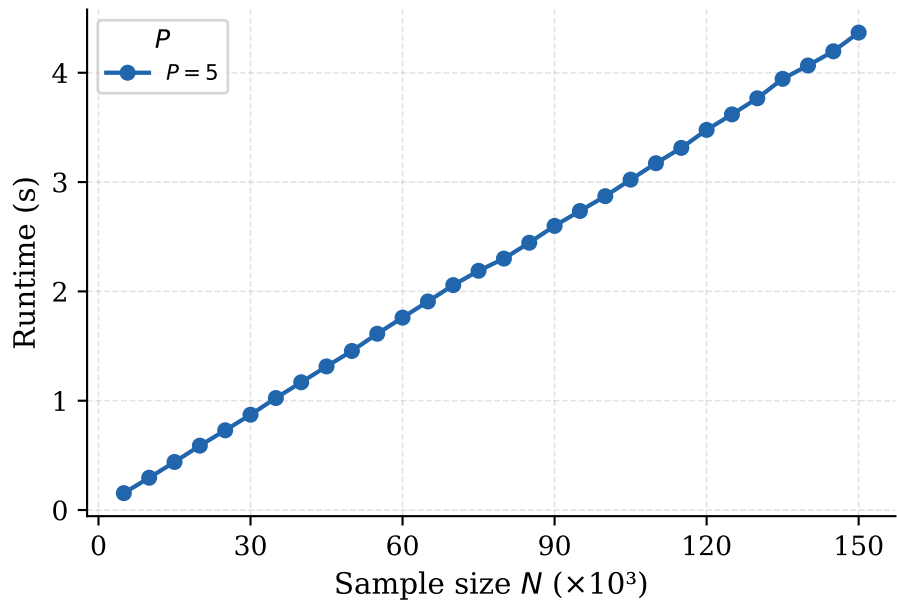
Gradient ascent
