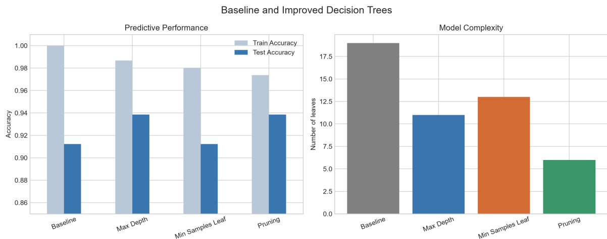
Hình 7.1: Trade-off giữa accuracy và số leaf của các mô hình
