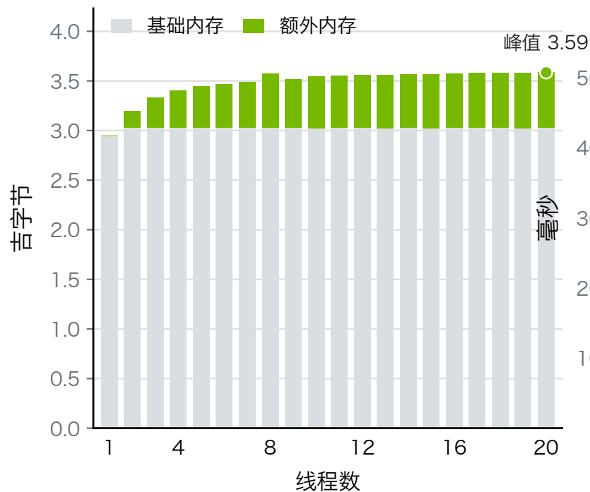
实测峰值内存
