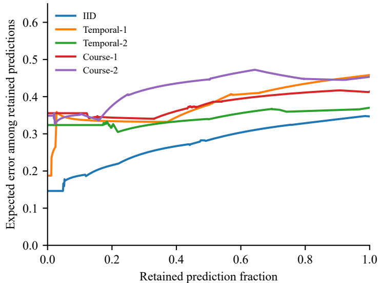
Catboost
