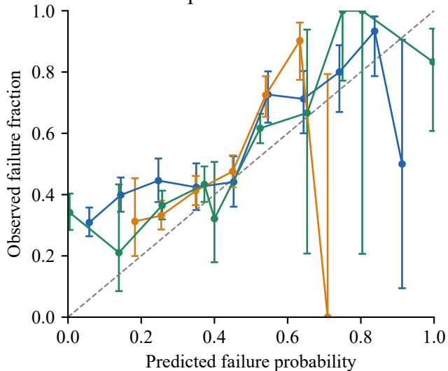
Temporal-2 / CatBoost
