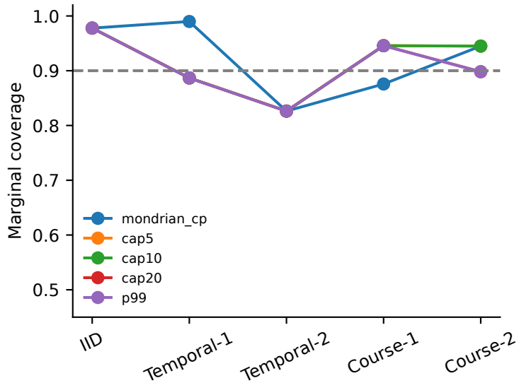
Catboost
