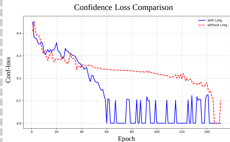
without L_{reg}
