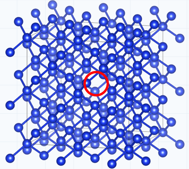
V_Si Vacancy
